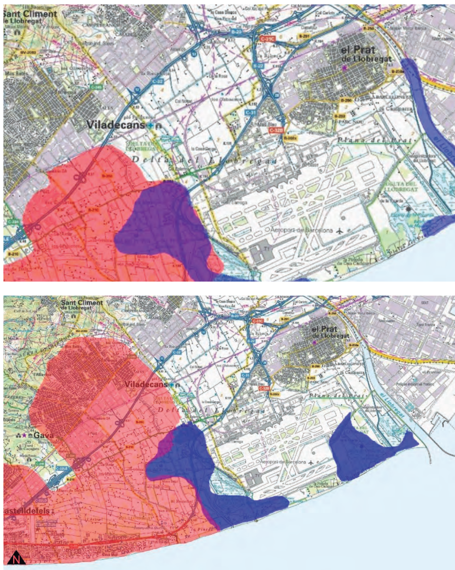
FIGURA 5. Àrees desfavorables respecte a l'amoni (vermell) i la conductivitat (blau) per a Epidaleia calamita (a dalt) i per a Pelophylax perezi (a baix). Font: PICMA del Consorci per a la Protecció i la Gestió dels Espais Naturals del Delta del Llobregat.
