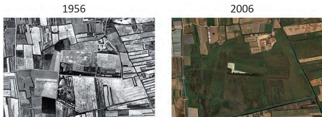
FIGURA 2. Aspecte del paratge dels Reguerons el 1956, quan era objecte d'explotació agrícola, i el 2006, ja abandonat i dominat per canyissars i jonqueres secundàries. La làmina d'aigua del centre correspon a una antiga explotació d'àrids abandonada. Imatges: ortofotomapes de l'ICGC.
