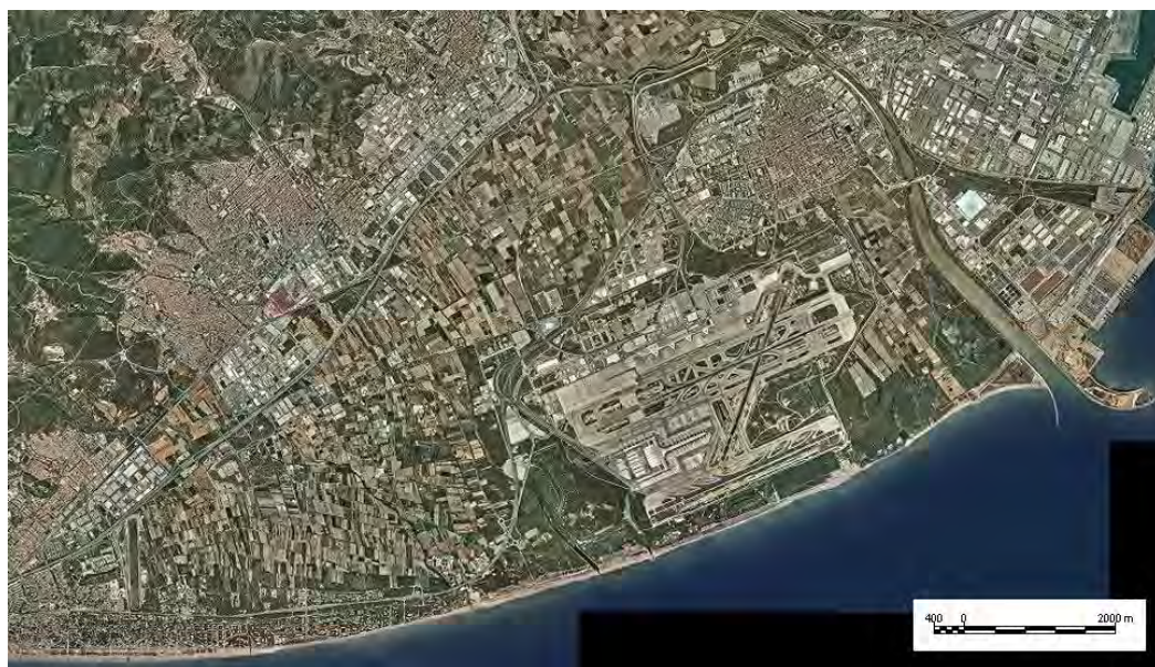
FIGURA 9. Fotografia aèria del delta del Llobregat, de l'any 2015. Font: ICGC.
