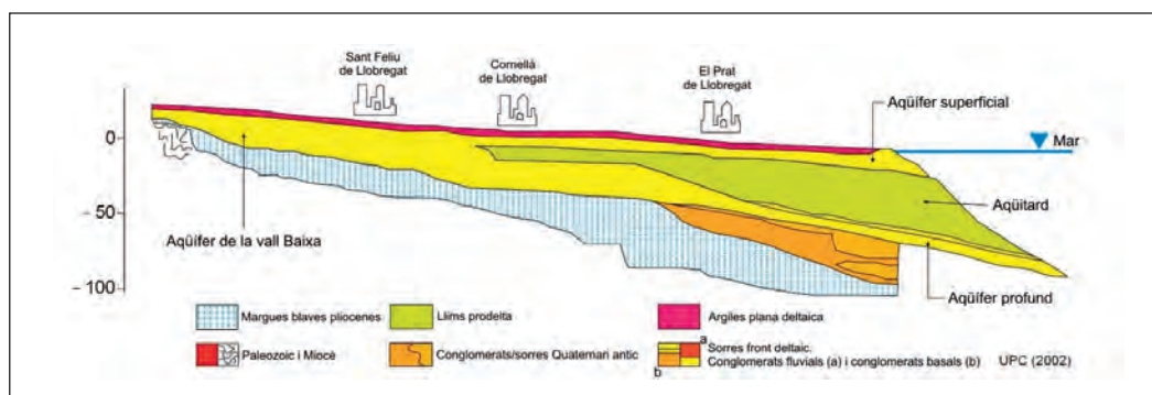
FIGURA 14. Tall longitudinal dels aqüífers de la vall Baixa i delta del Llobregat (Ministerio de Obras Públicas, 1966; Manzano et al. , 1993; modificat per UPC, 2002).
