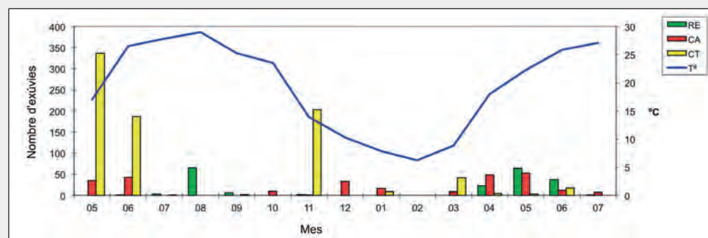
Variació mensual de la temperatura de l'aigua (°C) i del nombre d'exúvies (emergències d'adults) de quironòmids recollides en tres llacunes del delta del Llobregat (el Remolar: RE, Ca l'Arana: CA, Cal Tet: CT) entre maig-2004 i juliol-2005. Dades inèdites de Sánchez-Millaruelo, Cañedo-Argüelles i Rieradevall.
