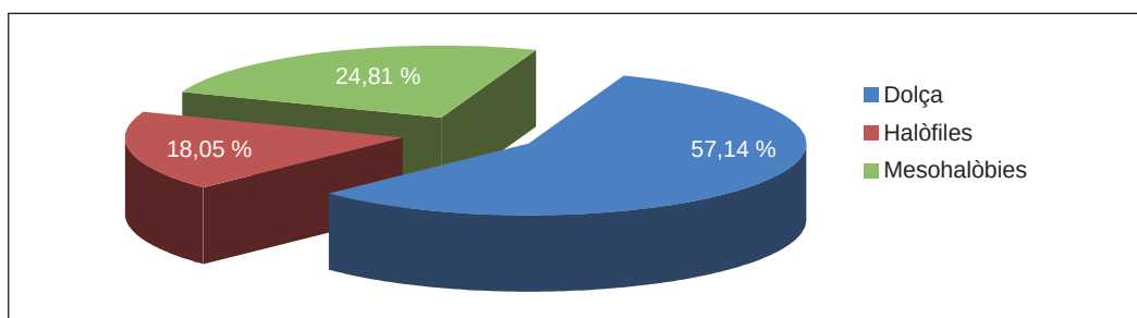
FIGURA 6. Preferències ecològiques respecte a la conductivitat de l'aigua de les algues identificades. Dades pròpies i diverses fonts mencionades a l'inici de l'apartat 5.2.
